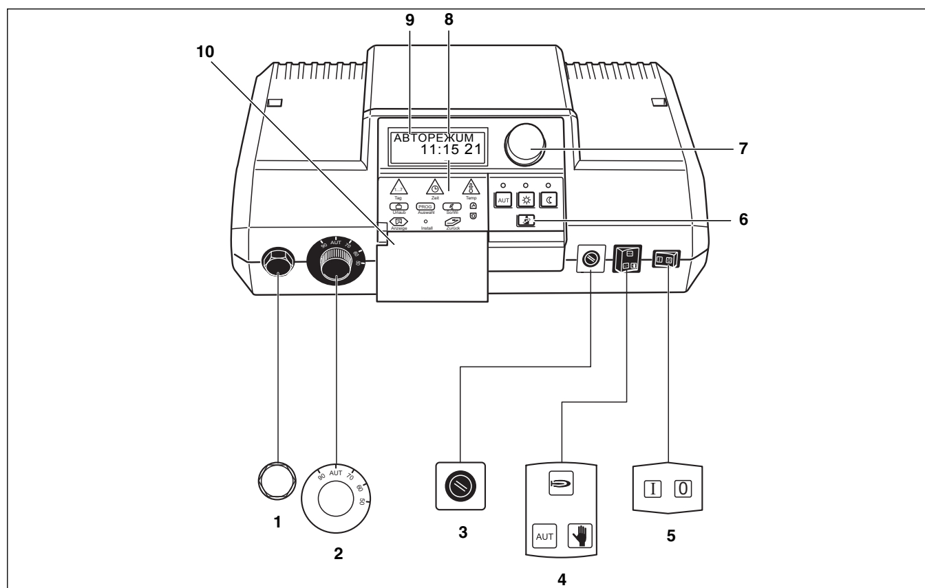
Рис. 1 Элементы управления Logamatic 2107 и Logamatic 2107 M
